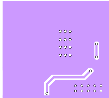
Bottom Layer
